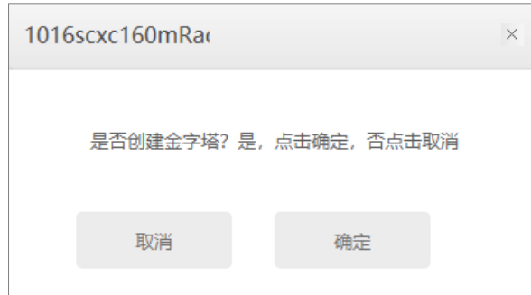
图 2-3 金字塔提示
