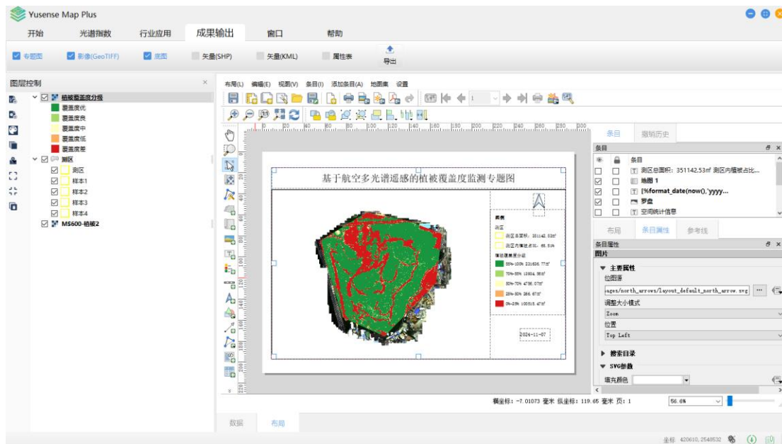
图 3-11 数据视图
