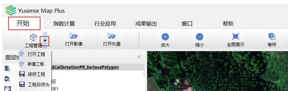
图 4-15 新建工程
