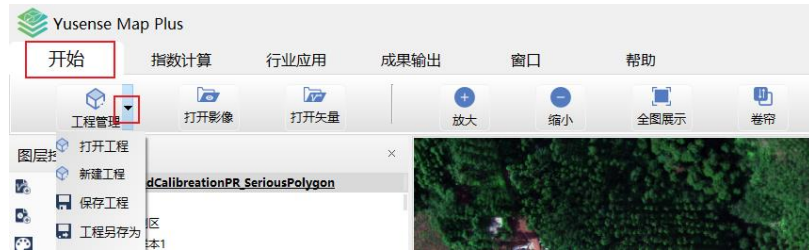
图 2-17 新建工程
