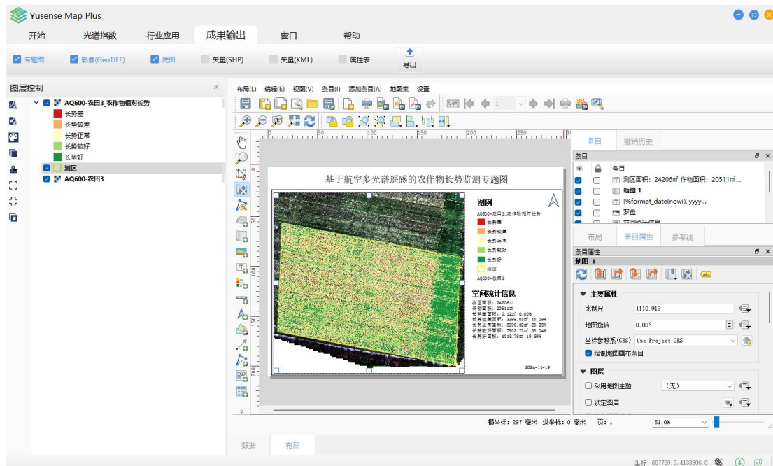
图 2-15 布局视图
