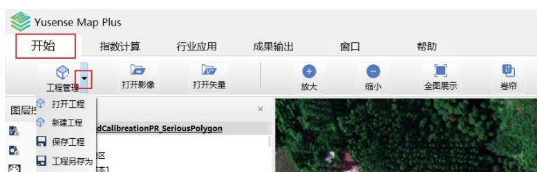
图 3-13 新建工程
