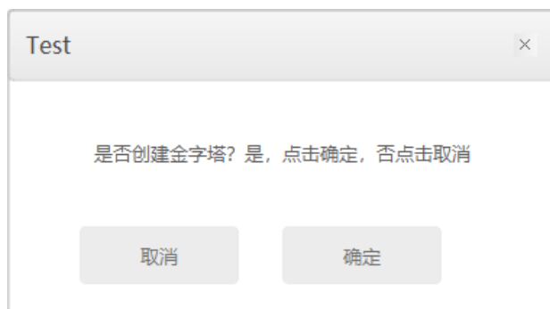
图 4-3 金字塔提示
